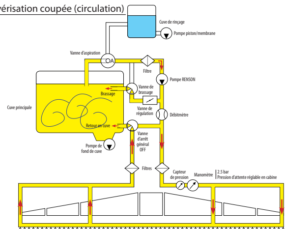
En pulvérisation - jets ouverts
