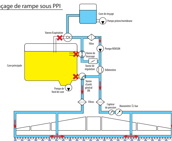
Rinçage de rampe sous PPI
